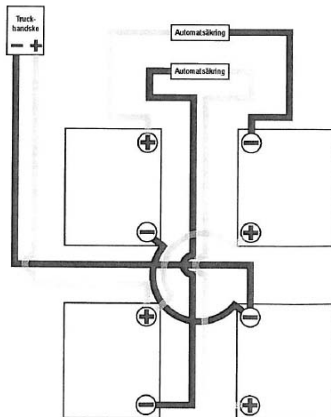
Principskiss 2 för anslutning av batterier
