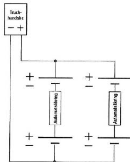
Principskiss 1 för anslutning av batterier
