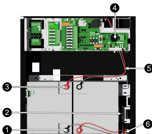
Figur 2. Moderkort kan skilja sig beroende på konfiguration men inkoppling av batterier sker på samma sätt.
