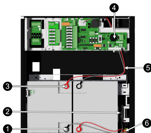
Figur 2. Hovedkortet kan variere avhengig av konfigurasjon, men tilkobling av batterier gjøres på samme måte.
