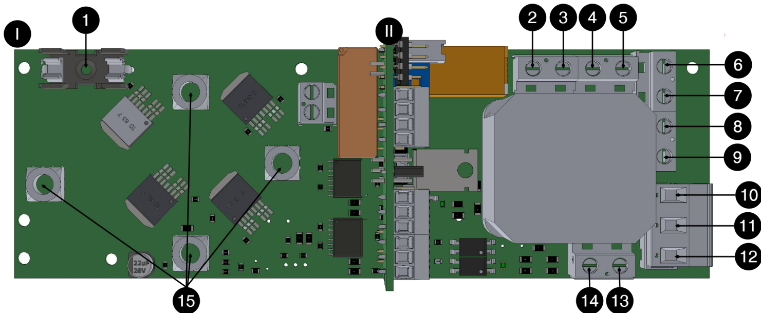
Piirilevyn yleiskatsaus, selitys
