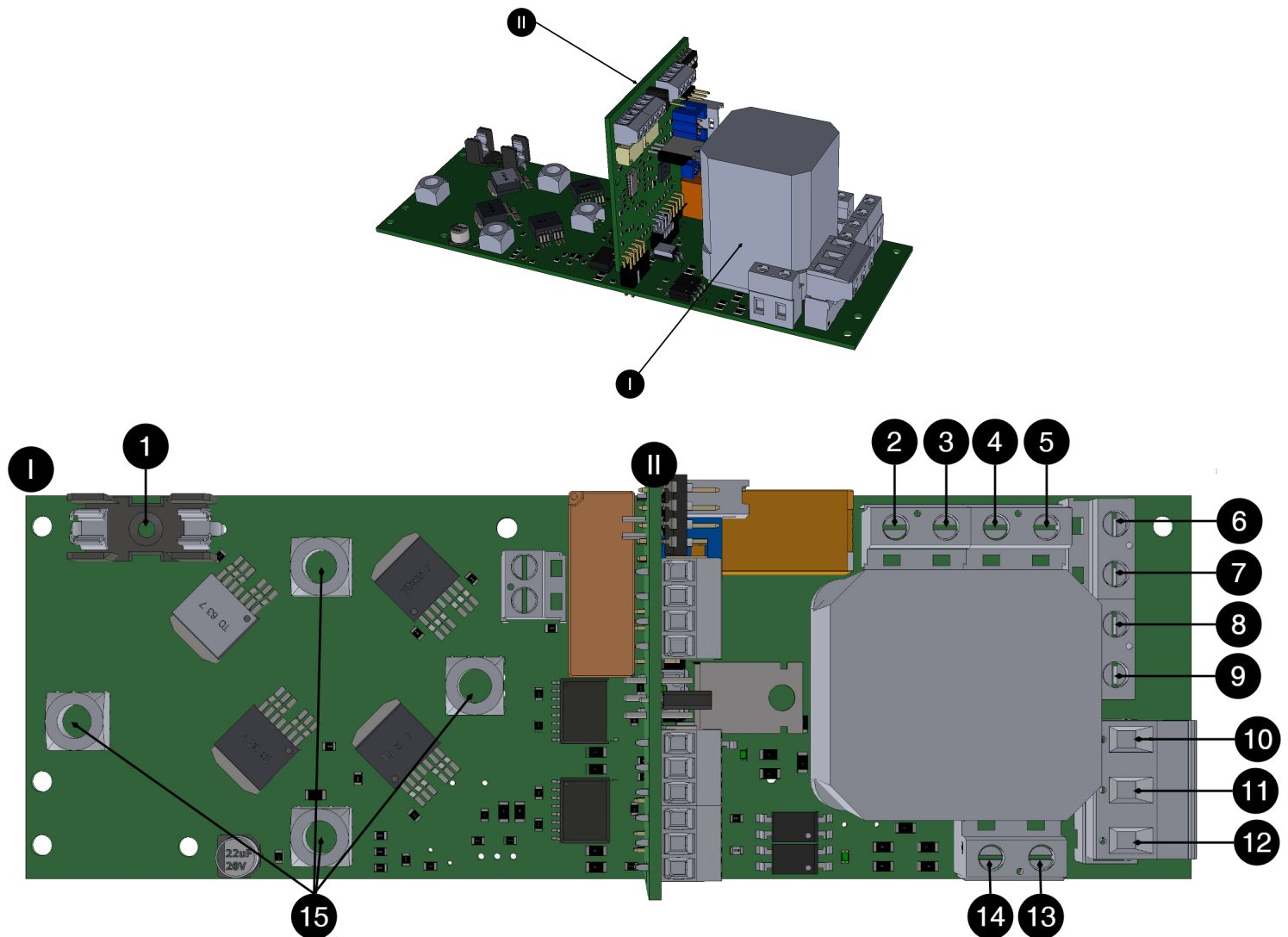
Kretskortoversikt, forklaring
