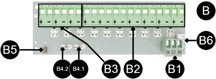
Kretskortoversikt 10 Utgangsmodul ATO -B: Bakside
