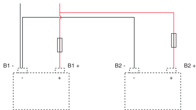
Parallellkoppling, batterier: 12 V
