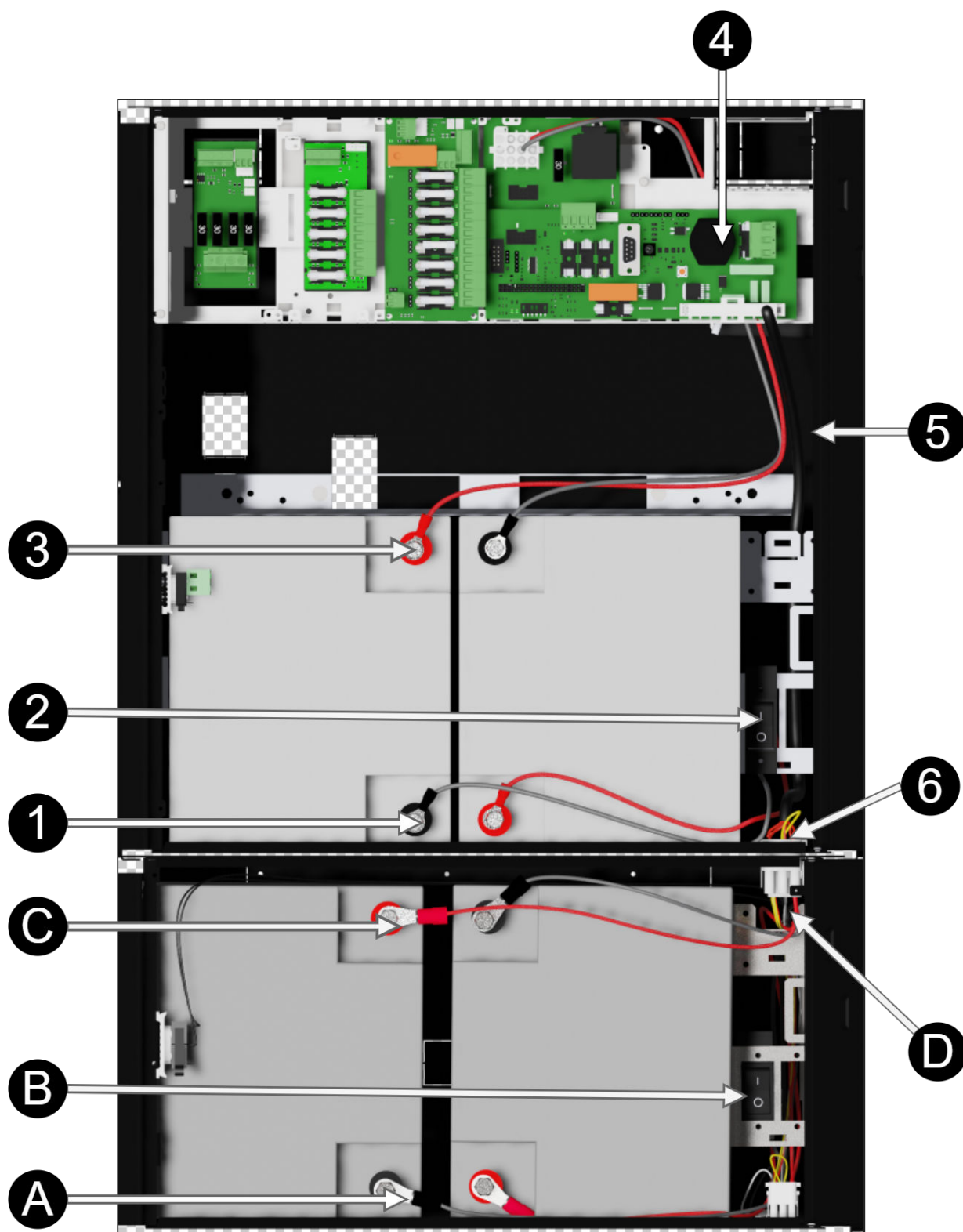
Figur 7. Moderkort kan skilja sig beroende på konfiguration men inkoppling av batterier sker på samma sätt.
