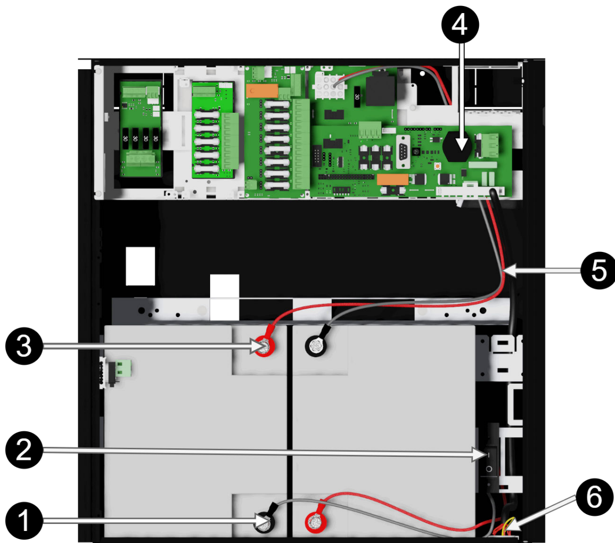
Figur 3. Moderkort kan skilja sig beroende på konfiguration men inkoppling av batterier sker på samma sätt.
