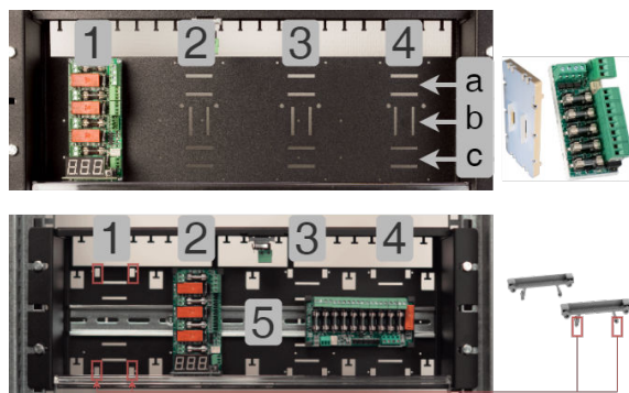
Figur 1. 19 rack module holder med olika kort monterade.
