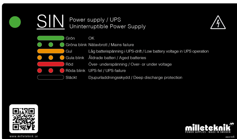
Panel för UPS med Minisinus i FLX M- och FLX L-koppling
