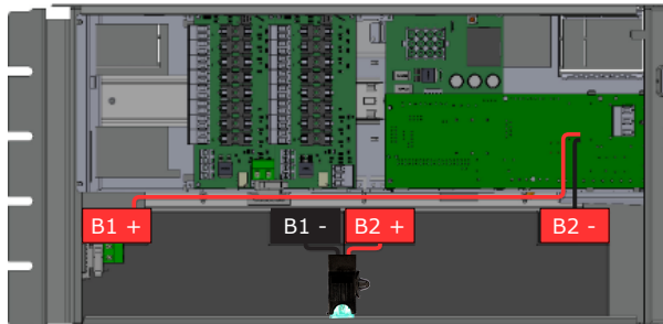
Seriokoppling, batterier: 24 V FLX M
