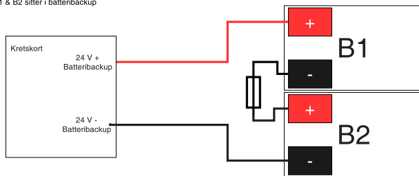
Seriokoppling, batterier: 24 V
