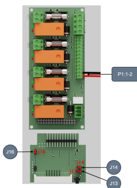
Exempel ett - Negativ logik - gemensam styrning (fabriksinställning).
