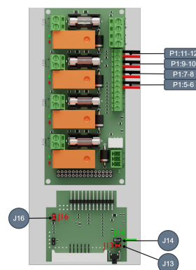
Exempel två: Negativ logik - individuell styrning.
