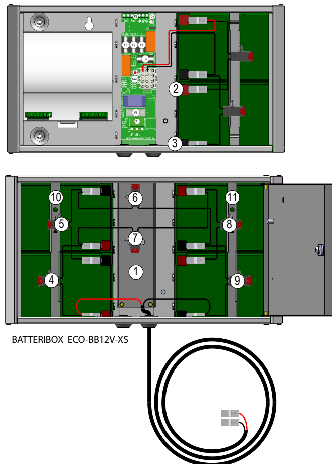
BEFINTLIG LIKRIKTARE (ECO 12V visad)
