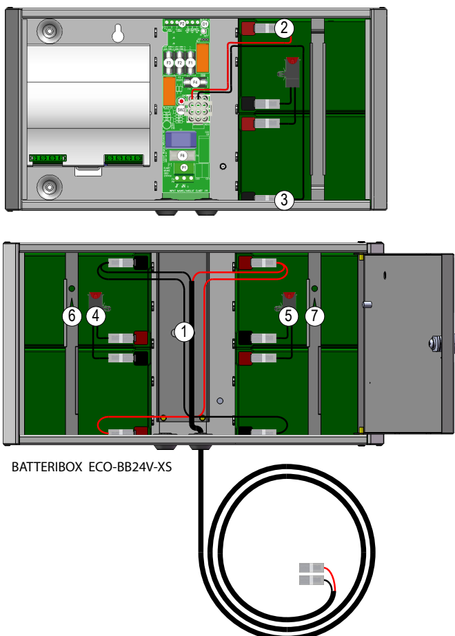
BEFINTLIG LIKRIKTARE (ECO 24V visad)
