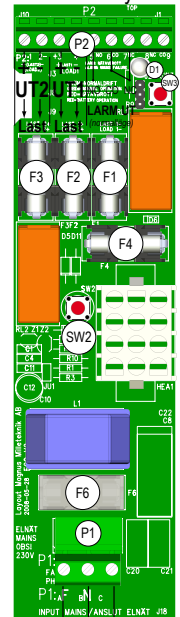
Kretskort ECOsystem
