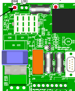
Kretskort BASsystem
